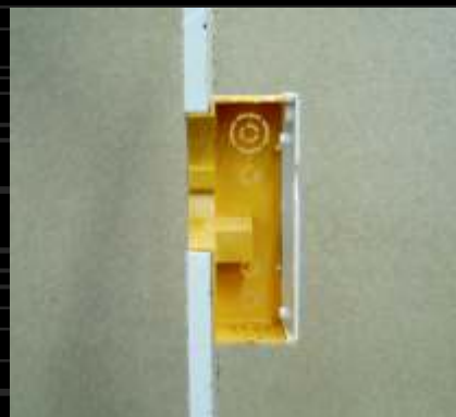
3) Boční pohled (v řezu) na krabici vloženou z rubové strany sádkartonové desky.
